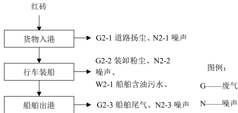
图 4-2 项目工艺流程及产污节点图（出货）
