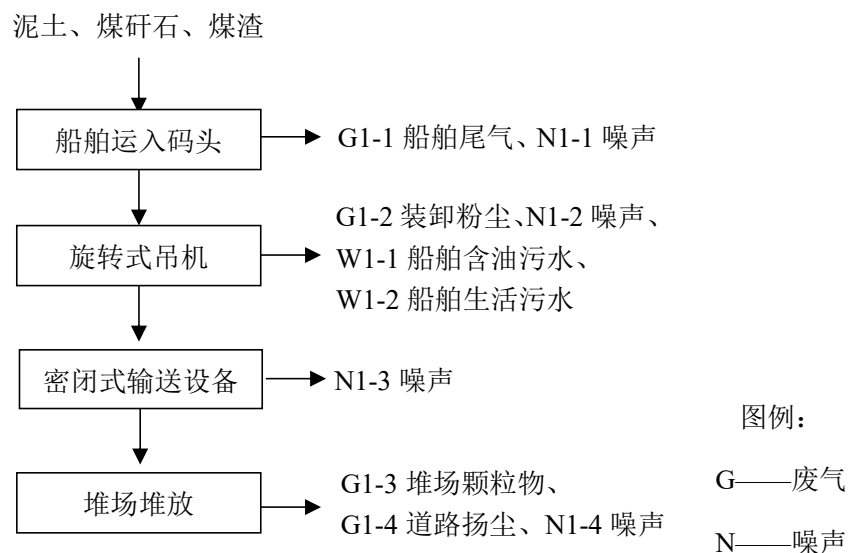
图 4-1 项目工艺流程及产污节点图（进料）
