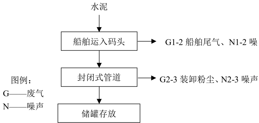
图 4-2 项目工艺流程及产污节点图
