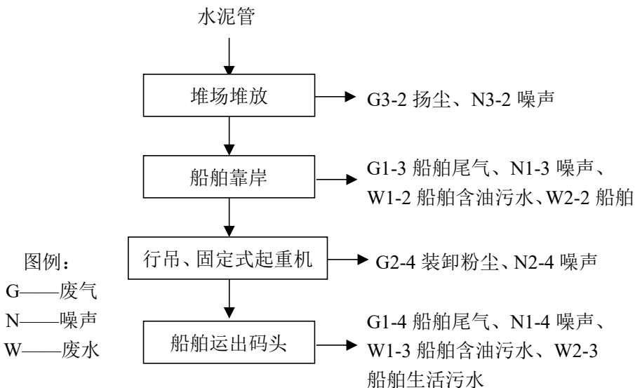
图 4-3 项目工艺流程及产污节点图
