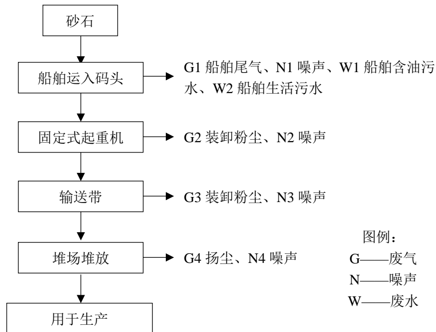
图 4-1 项目工艺流程及产污节点图
