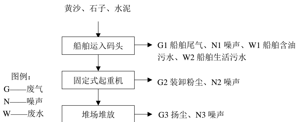
图 4-1 项目工艺流程及产污节点图
