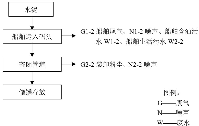
图 4-2 项目工艺流程及产污节点图
