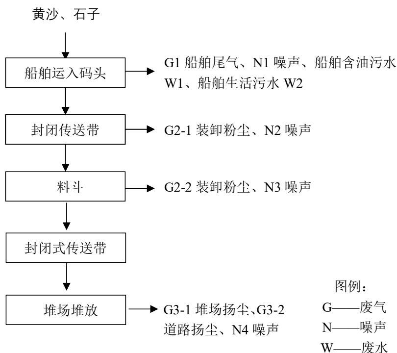
图 4-1 项目工艺流程及产污节点图
